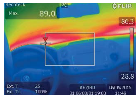
Innenraumaufnahme VW Tiguan schwarz, mit Wärmeschutzfolie, mit Wärmebildkamera.
