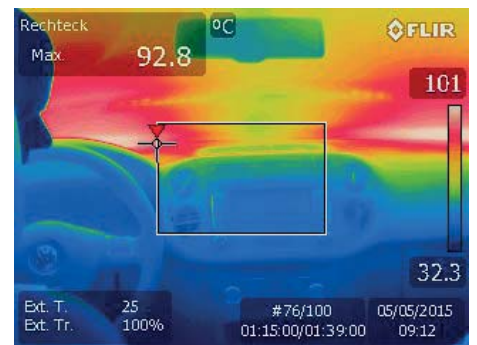
Innenraumaufnahme VW Tiguan schwarz, 3 cm Fenster offen, mit Wärmebildkamera.
